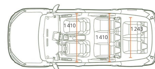
VUE DE DESSUS 7 PLACES
